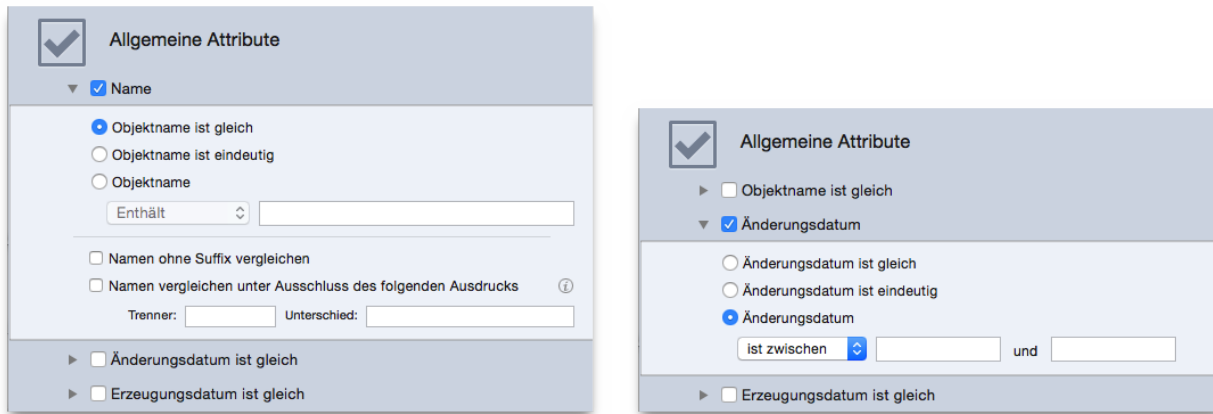
Abb. 17: Allgemeine Attribute.
