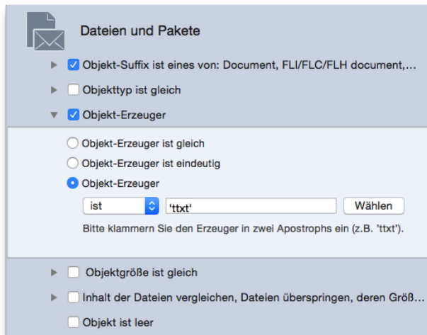
Abb. 21: Abschnitt Objekt-Erzeuger-Suchkriterien.
