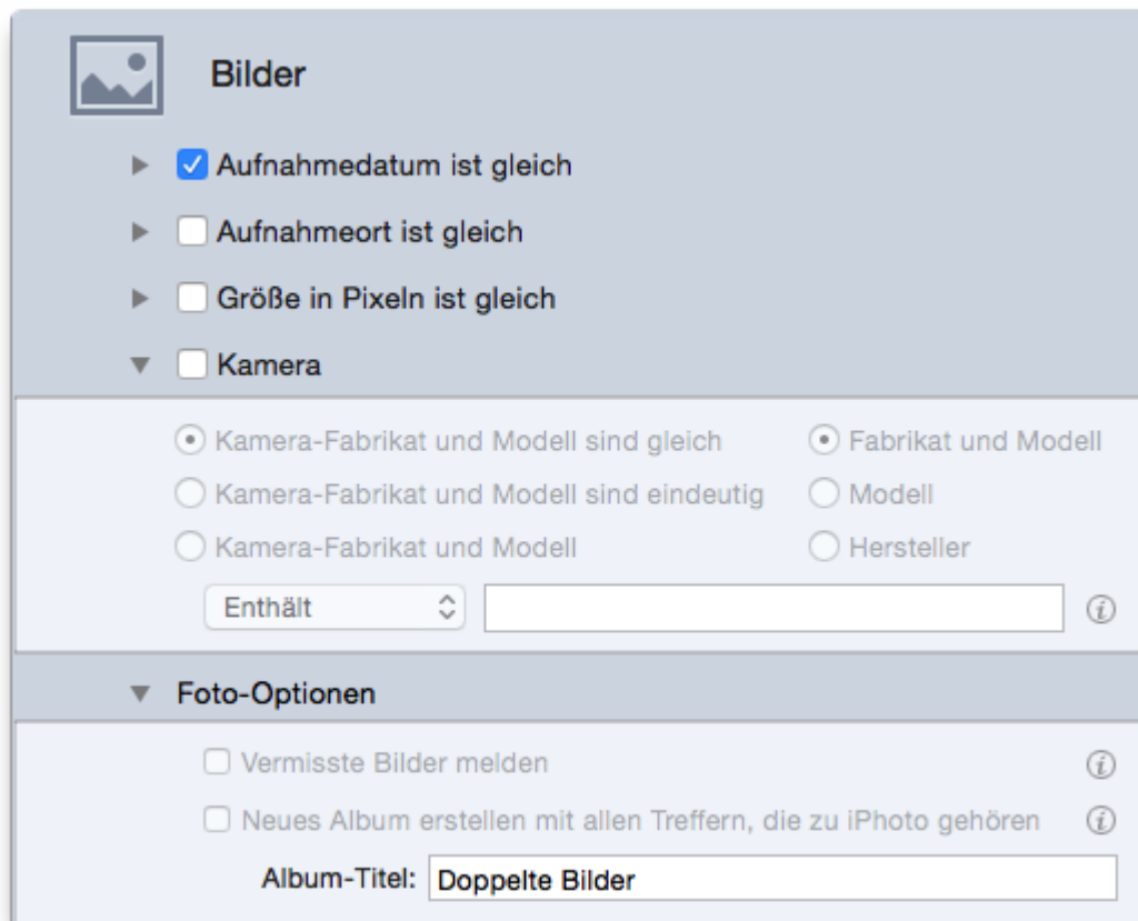
Abb. 29: Suchkriterienfeld Bilder.
