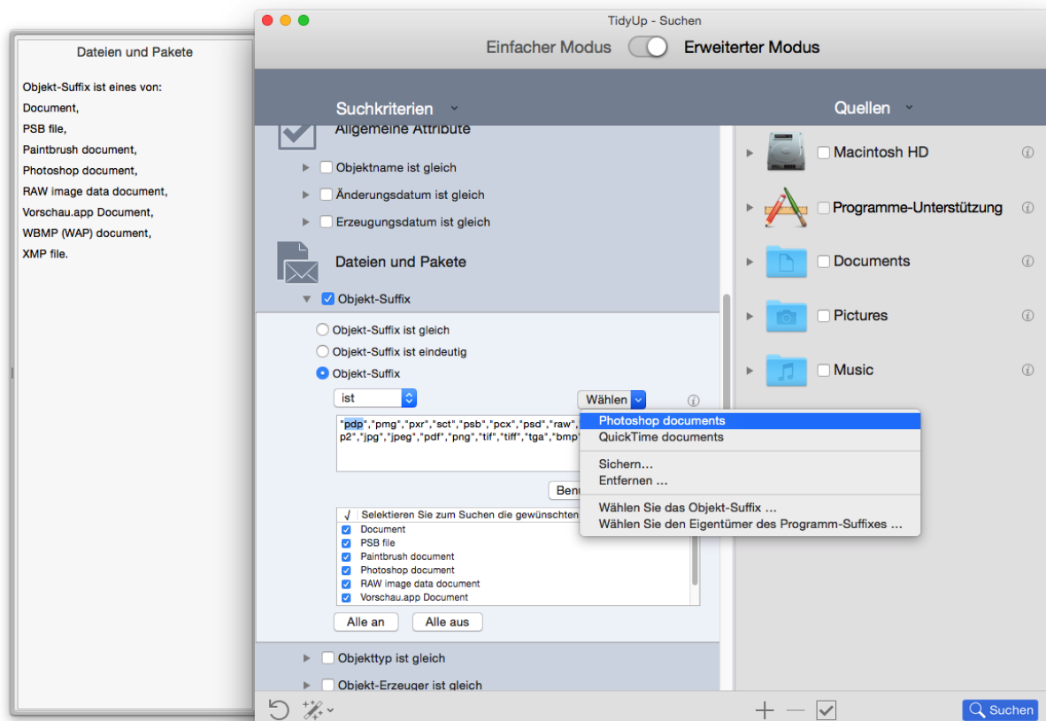
Abb. 19: Abschnitt Objekt-Endung-Suchkriterien.
