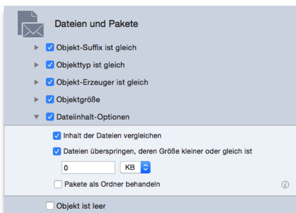
Abb. 23: Abschnitt Dateiinhalt-Suchkriterien.
