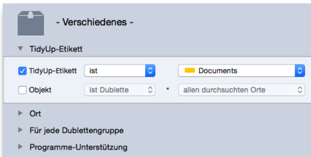
Abb. 52: TidyUp-Etikett.
