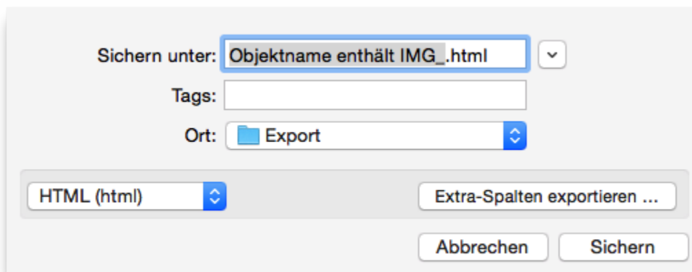
Abb. 70: Exportieren-Fenster.
