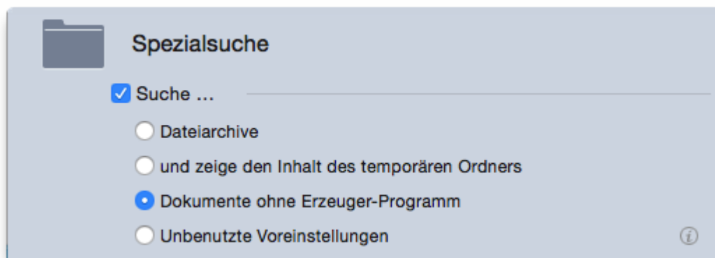
Abb. 30: Suchkriterienfeld Spezielsuche.
